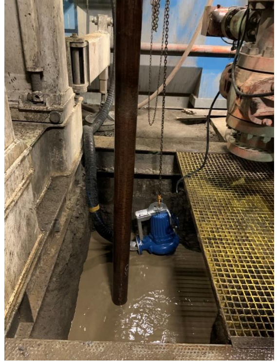
图4: 井口
